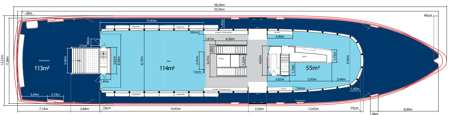
Hauptdeck
