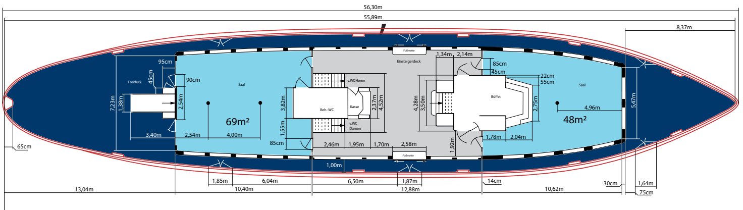
Hauptdeck
