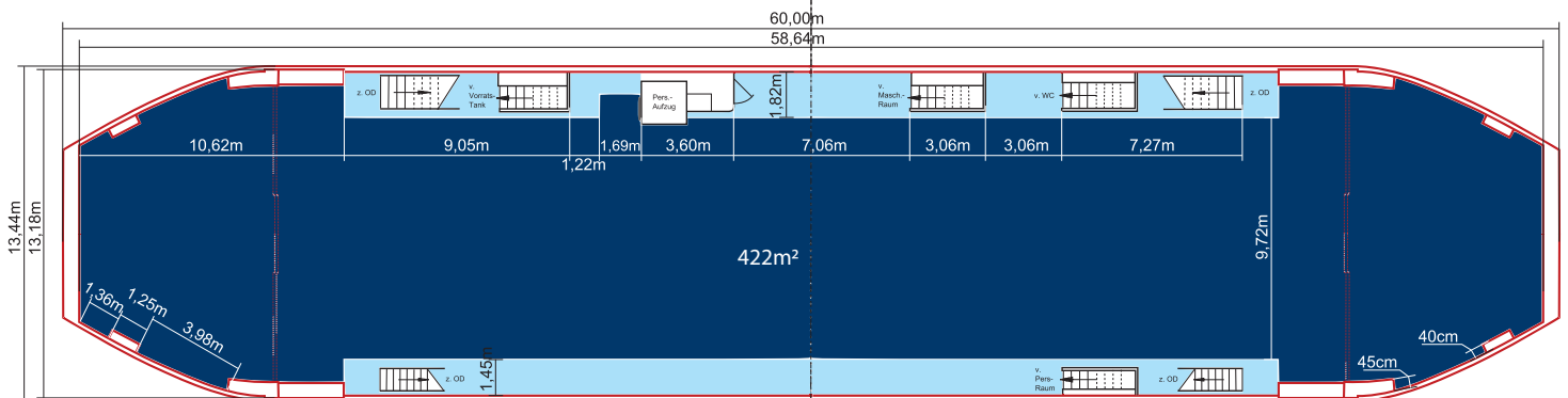
Hauptdeck
